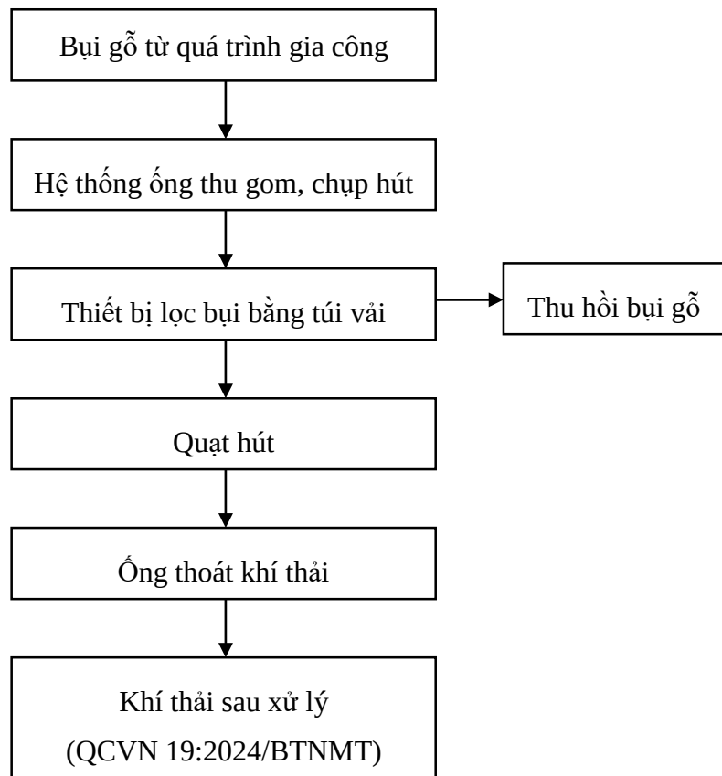
Hình 3.6. Sơ đồ công nghệ hệ thống xử lý khí thải bụi công suất 150.000\text{ m}^3/\text{giờ}
