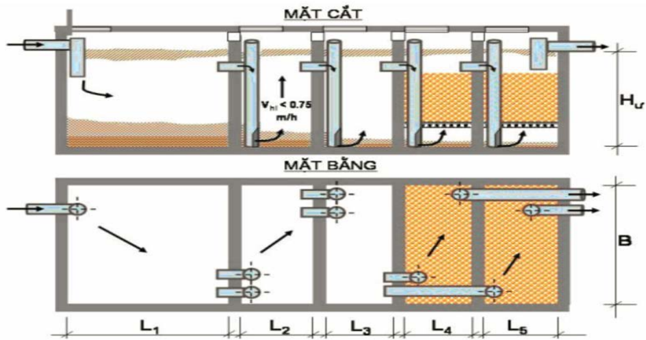
Hình 3.5. Minh họa cấu tạo bể tự hoại 5 ngăn
