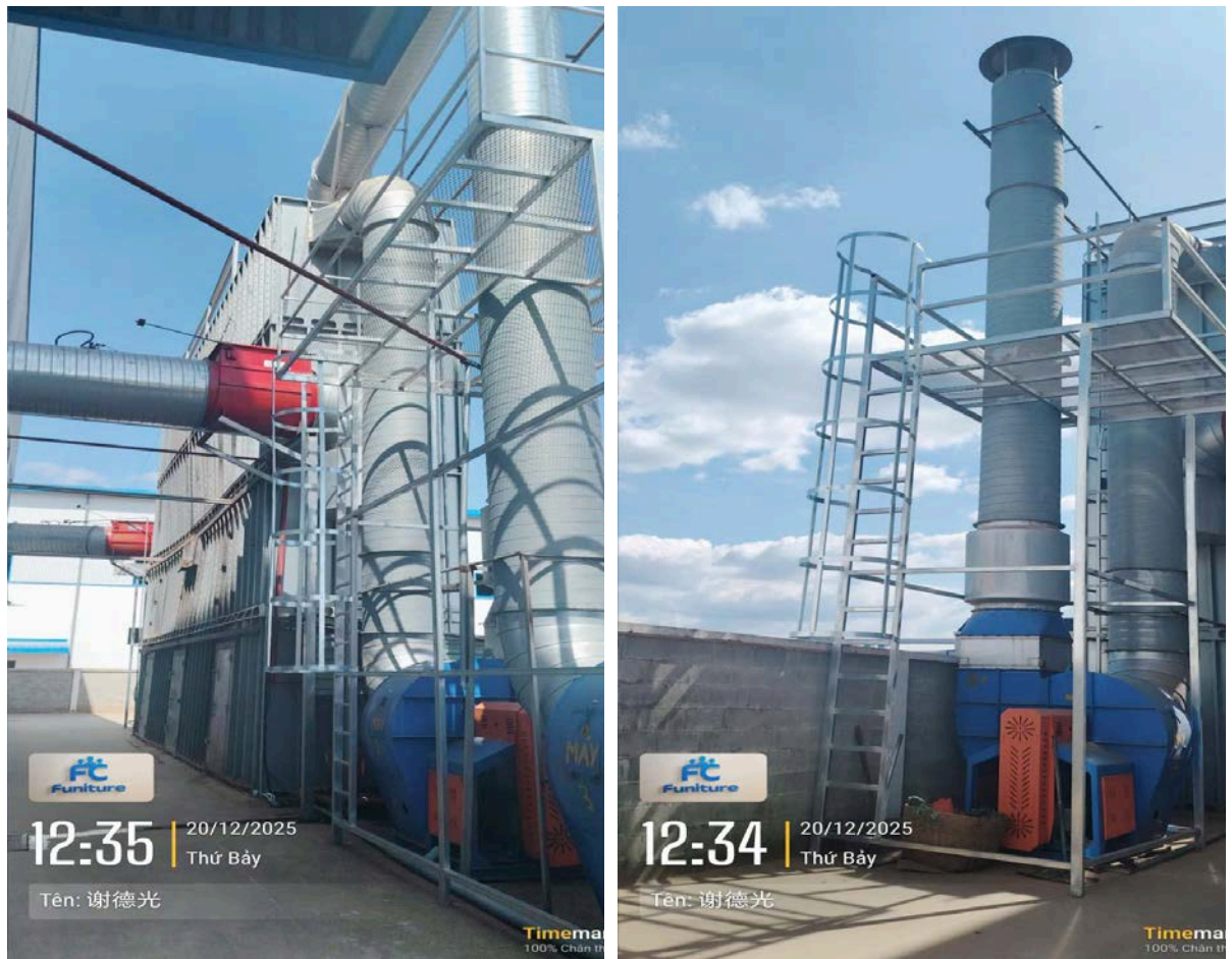
Hình 3.7. Hệ thống xử lý khí thải bụi công suất 150.000 m 3 /giờ
