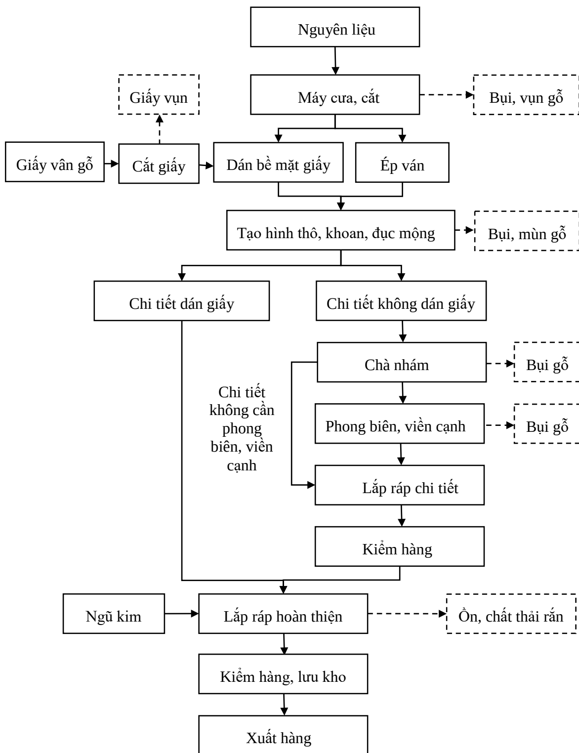
Hình 1.3. Quy trình công nghệ sản xuất của cơ sở
