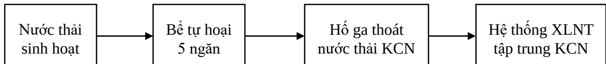
Hình 3.4. Sơ đồ hệ thống thu gom, thoát nước thải
