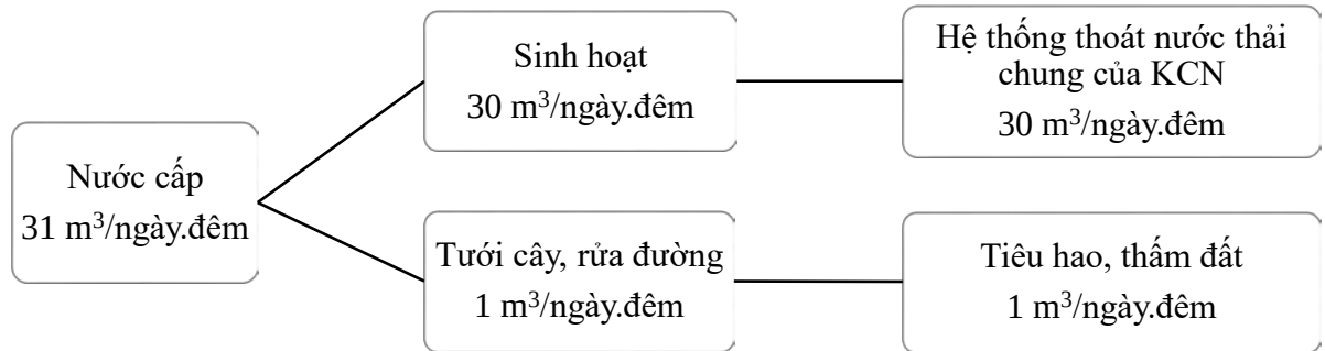
Hình 1.15. Sơ đồ cân bằng nước tại cơ sở
